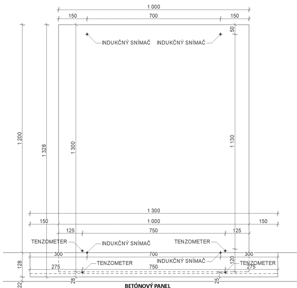
Schéma zostavy AL0009
