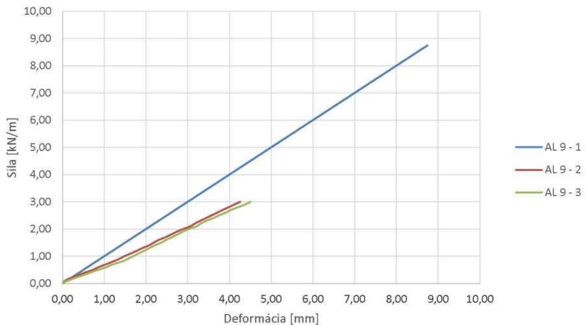
Graph der Abhängigkeit der Formänderung der Oberkante des Profils von der Kraft
