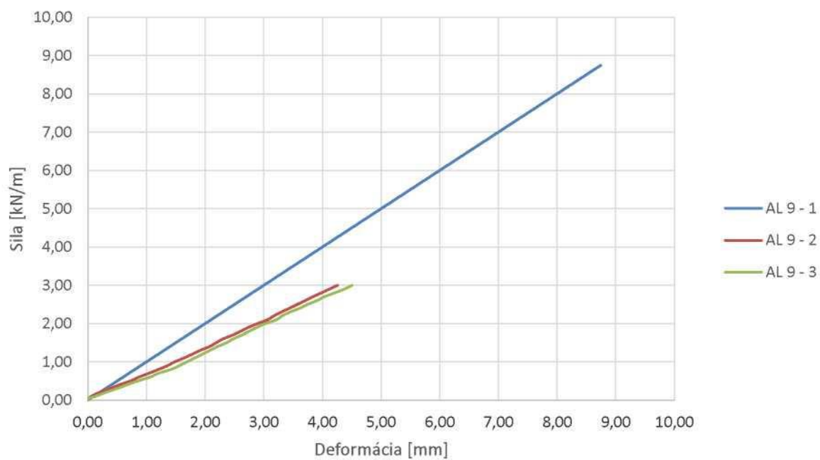
Graf závislosti pretvorenia hornej hrany profilu na sile
