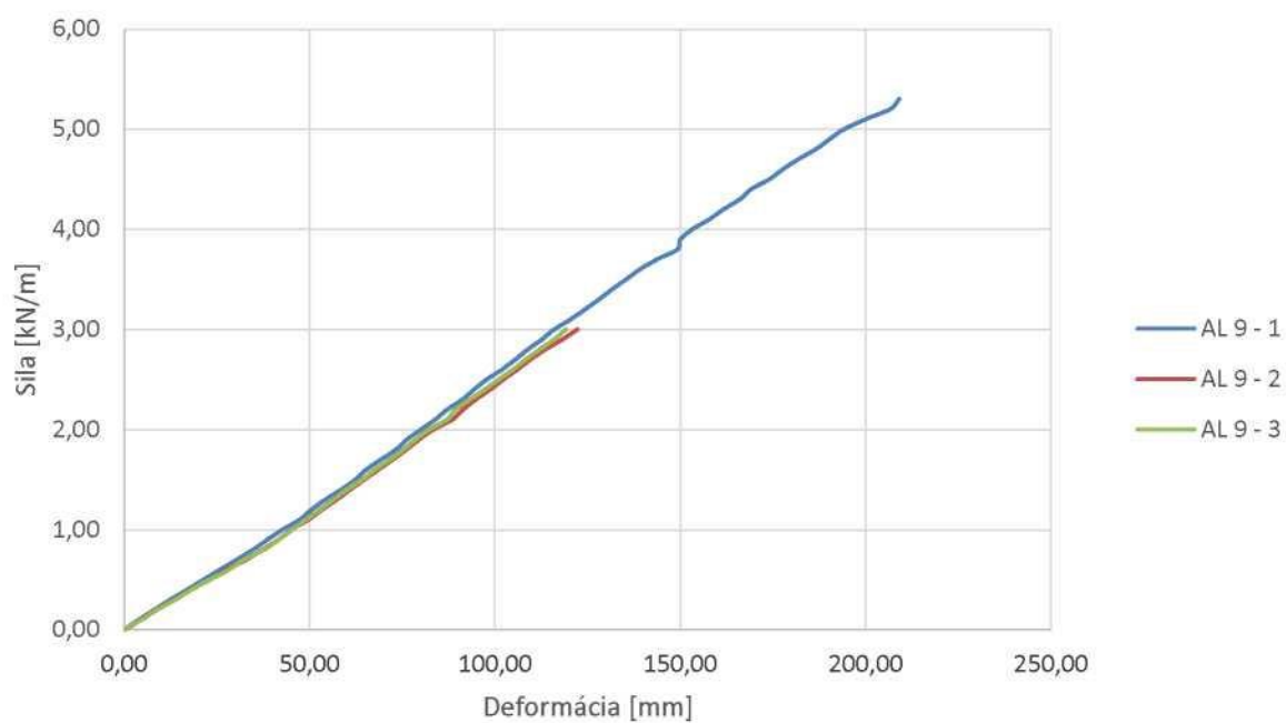
Graf závislosti pretvorenia skla na sile
