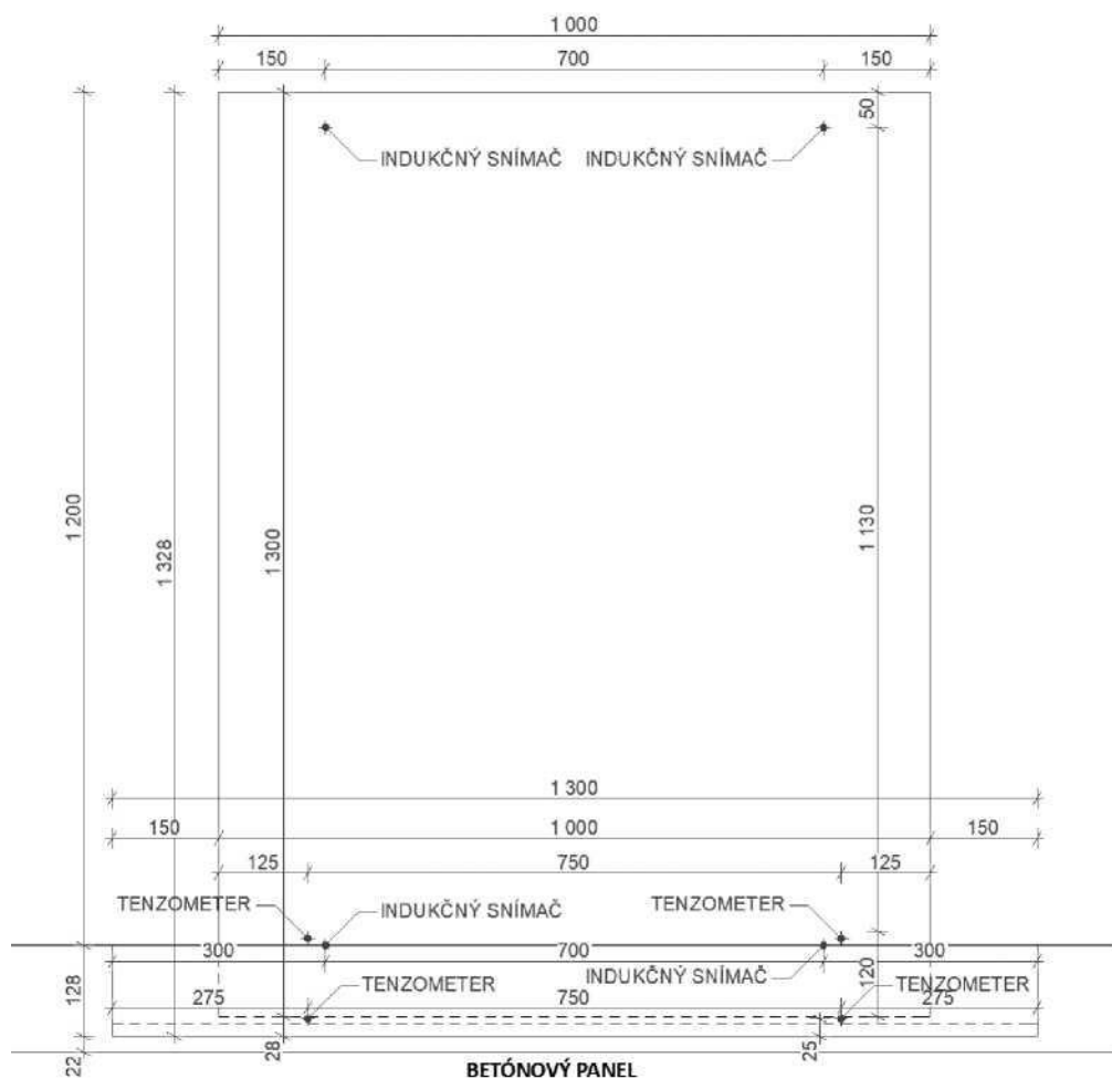
Schemat zestawu AL0009
