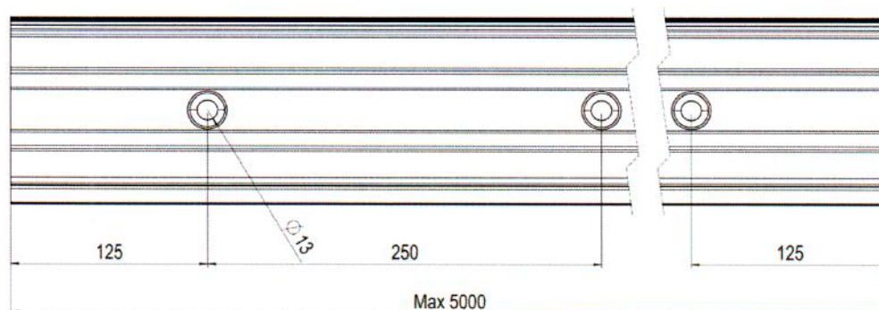
Abb. 2: Grundprofil AL/0005-5000-D-S-E Befestigung seitlich
