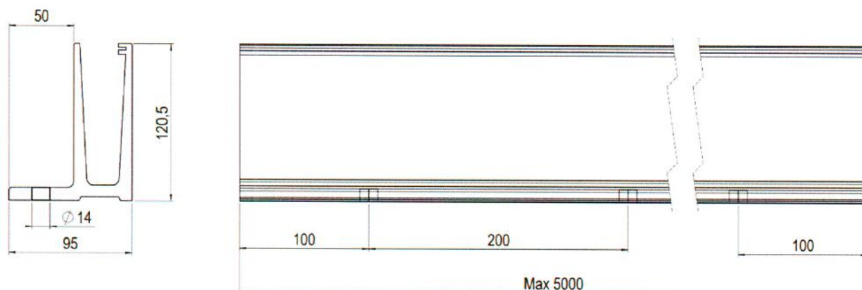
Abb. 4: Grundprofil AL/0006-5000-S-E Befestigung von oben
