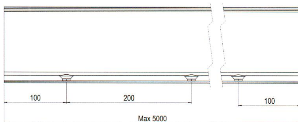
Abb. 1: Grundprofil AL/0004-5000-S-E Befestigung von oben
