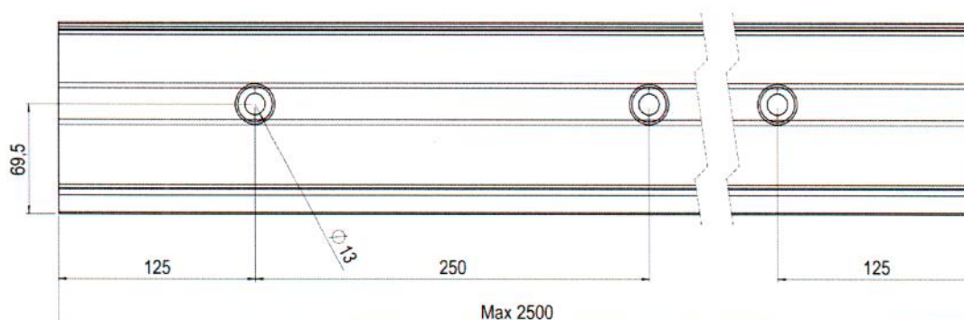
Abb. 3: Grundprofil AL/0005-2500-S-E Befestigung seitlich
