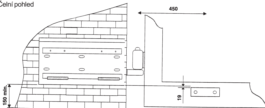
Čelní pohled
